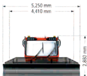
PistenBully 600
